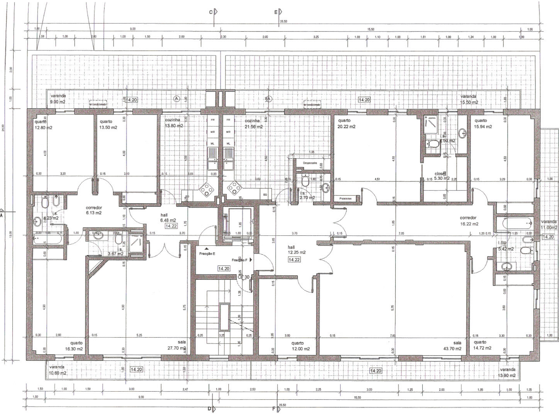
Planta do Piso 3
